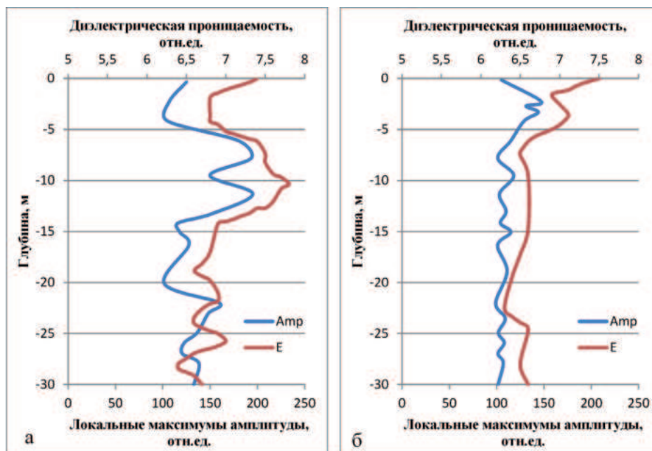
Рис. 3. Сопоставление значений диэлектрической проницаемости пород (E) и локальных максимумов амплитуд (Amp) огибающей электромагнитного сигнала по данным натуральных измерений: а – пятый метр профиля, б – двадцатый метр профиля.
