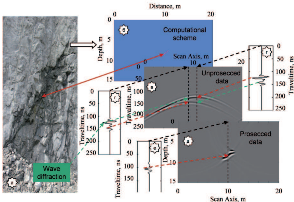
Рис. 1. Алгоритм и результаты моделирования электромагнитного поля, индуцируемого электромагнитным зондированием, в окрестности наклонной неоднородности.
