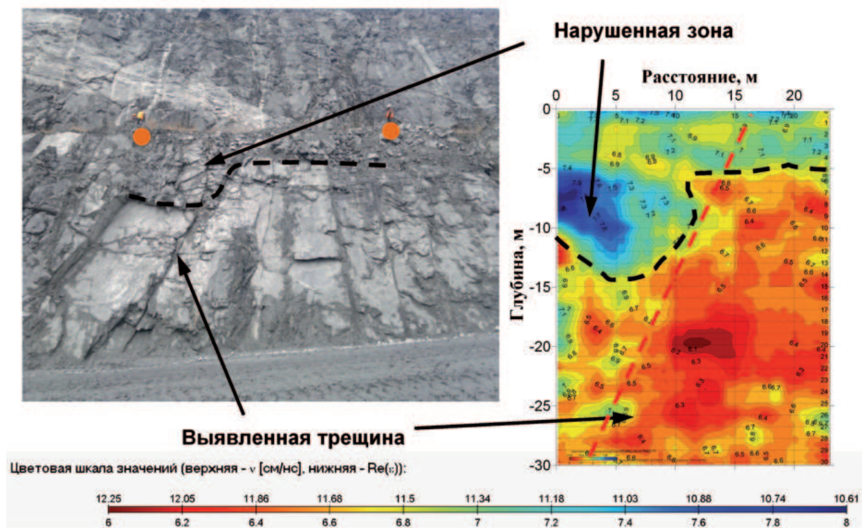
Рис. 2. Радарограмма и ее сопоставление с обнажением пород на уступе (начало и конец профиля обозначены на фото оранжевыми метками).
